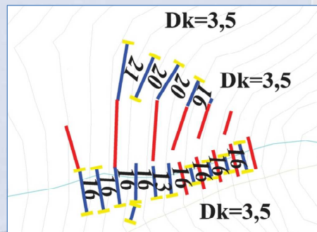
Planimetria di tracciamento "Rio del Larice" Linea blu: elementi intermedi "VELA-Fermaneve" Linea gialla: elementi marginali "VELA-Fermaneve"
