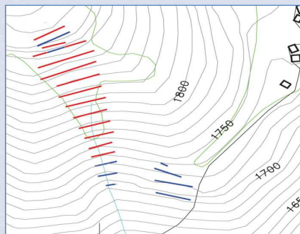
Planimetria di tracciamento "Piana dell'Orso" Linea blu: elementi "VELA-Fermaneve"
